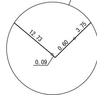
拡大図 S=50
