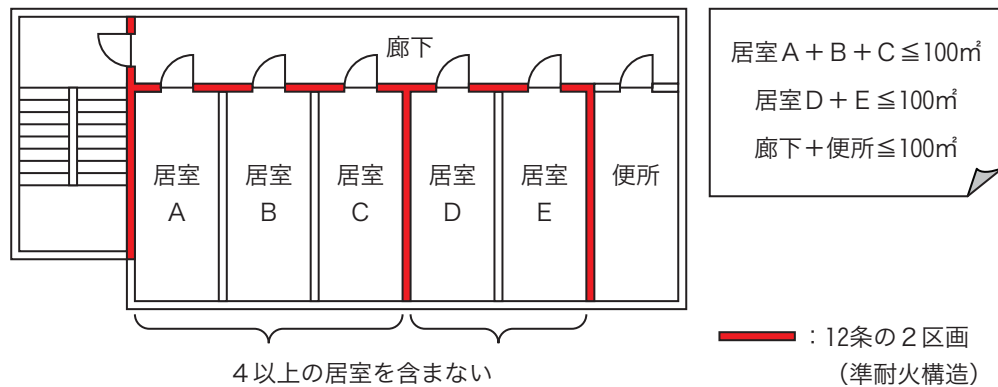
(2の階を一の12条の2区画する場合の例)
