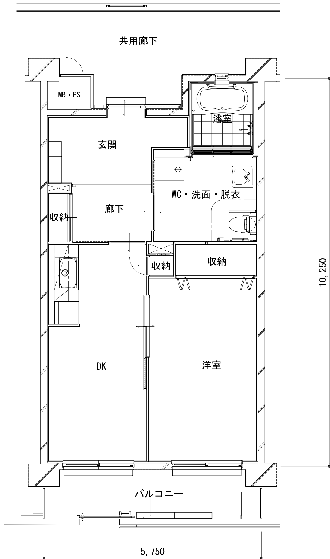
1DK身障者型平面図
