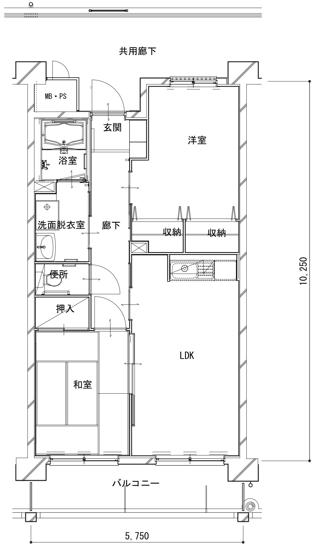
2LDK型平面図
