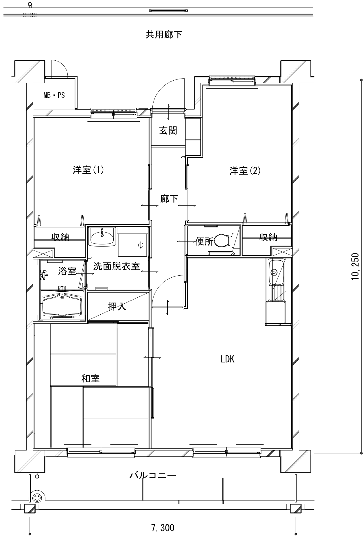
3LDK型平面図
