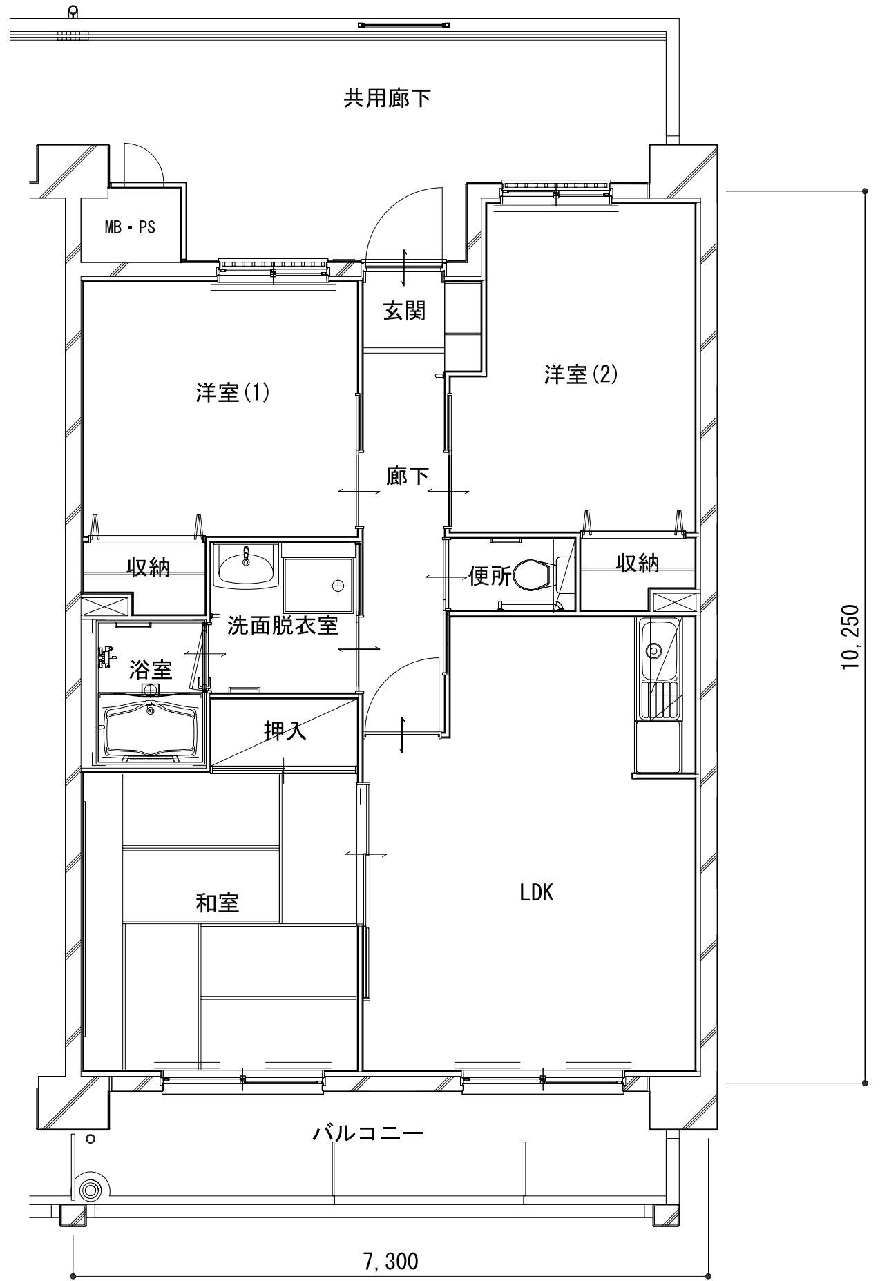
3LDK型(妻面)平面図
