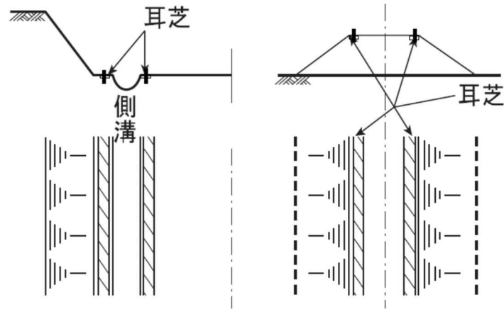
図3-2-6 耳 芝
