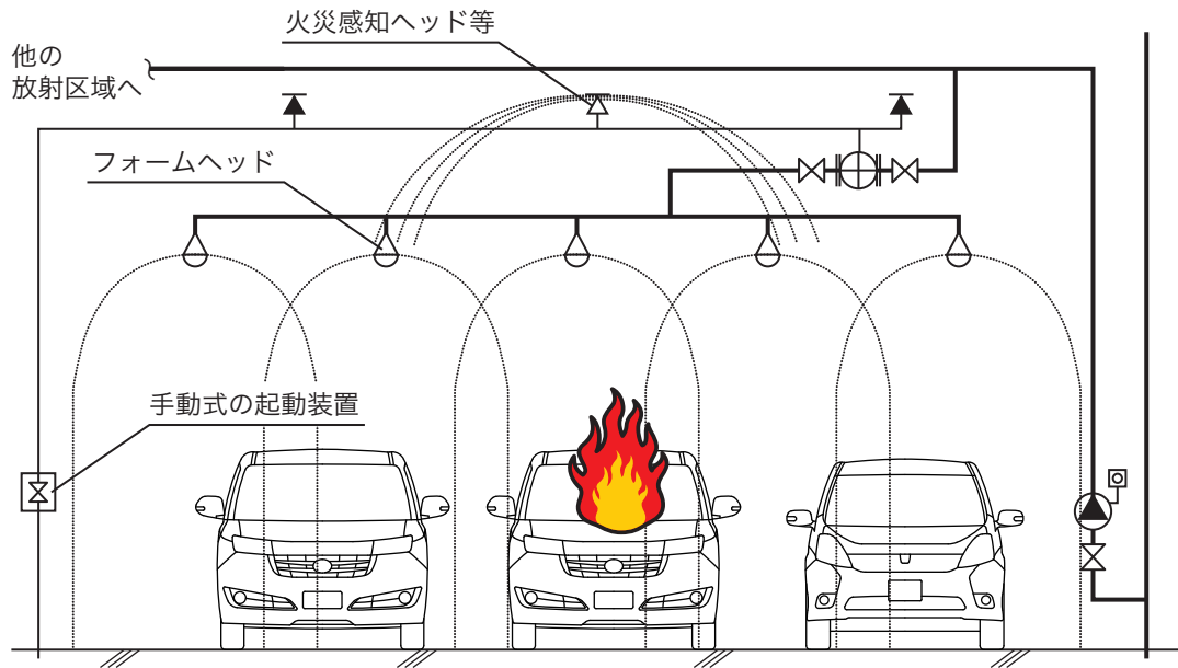
(泡消火設備の構成例)
