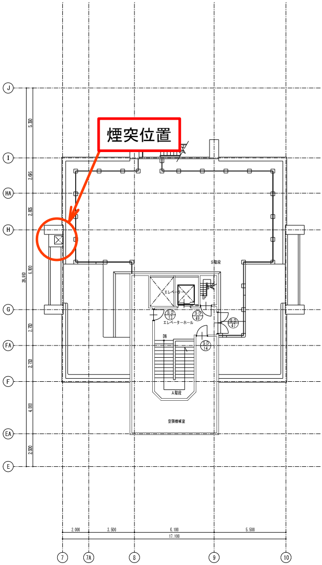
R階平面図 1:100
