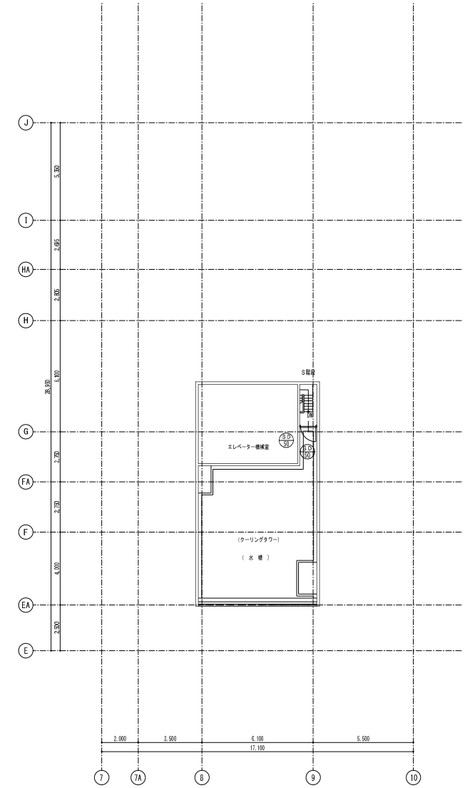
PH3階平面図 1:100
