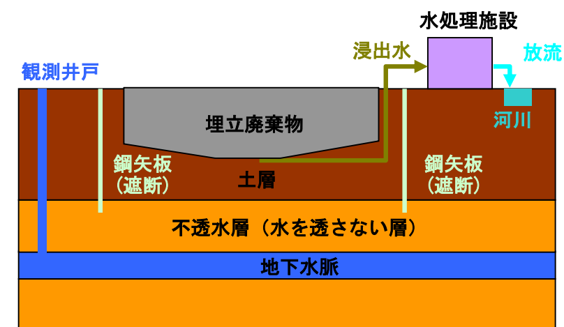
【埋立完了地の構造図】
