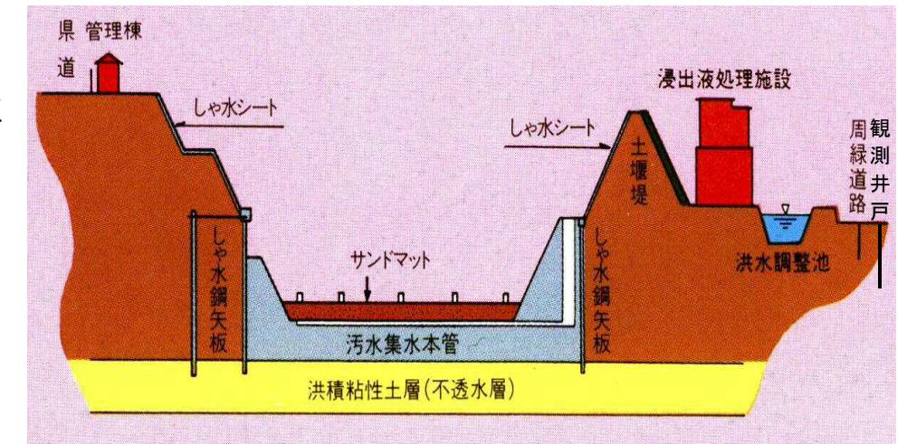
【最終処分場の構造図】
