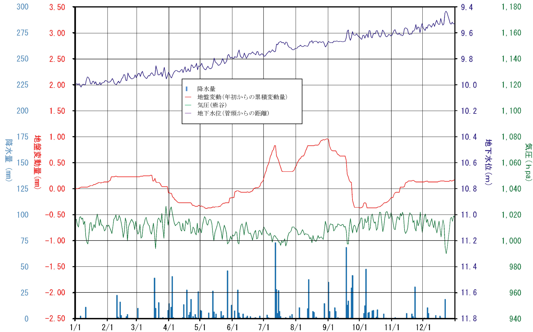
大宮観測所 地盤変動・地下水位変動図
