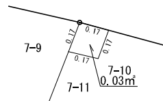
< 拡大図 >
