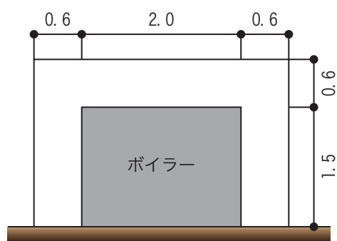
（立面図）
