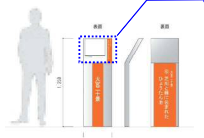
（表示板の拡大イメージ） 大宮区全体図の縮小版、現在地表示、当該二十景の解説文・写真、QRコードを記載 次ページ以降「個別案内板解説内容」参照
